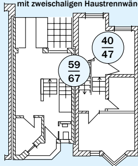
Doppel- und Reihenhäuser mit zweischaligen Haustrennwänden
